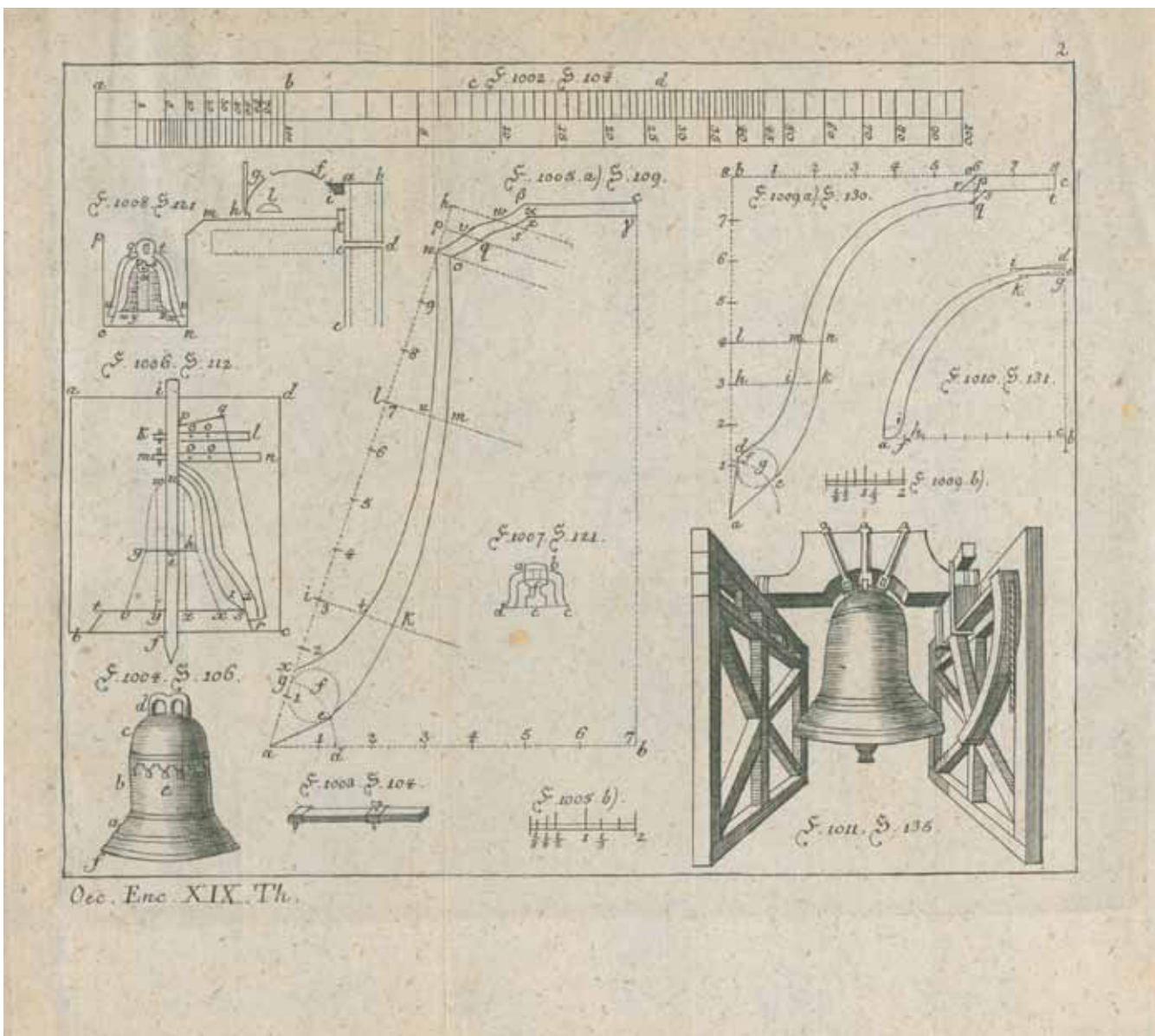
Darstellung des Herstellungsprozesses einer Glocke in Krünitz: Oekonomische Encyclopädie, 1780 (Staatsbibliothek zu Berlin, Abt. Hist. Drucke, Signatur Rara RLS Ae 2200 19) 1
